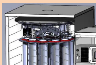
Sistema di pulizia caldaia automatico
