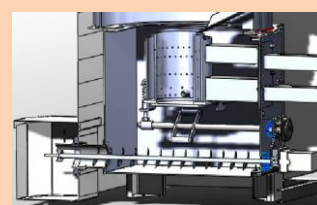
Sistema di pulizia del braciere automatico
